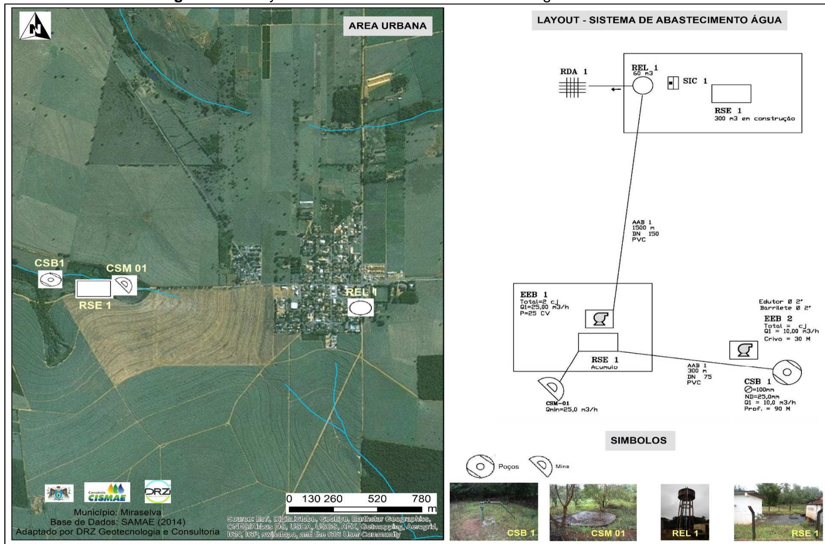
Figura 1.2 – Layout do sistema de abastecimento de água da área urbana
