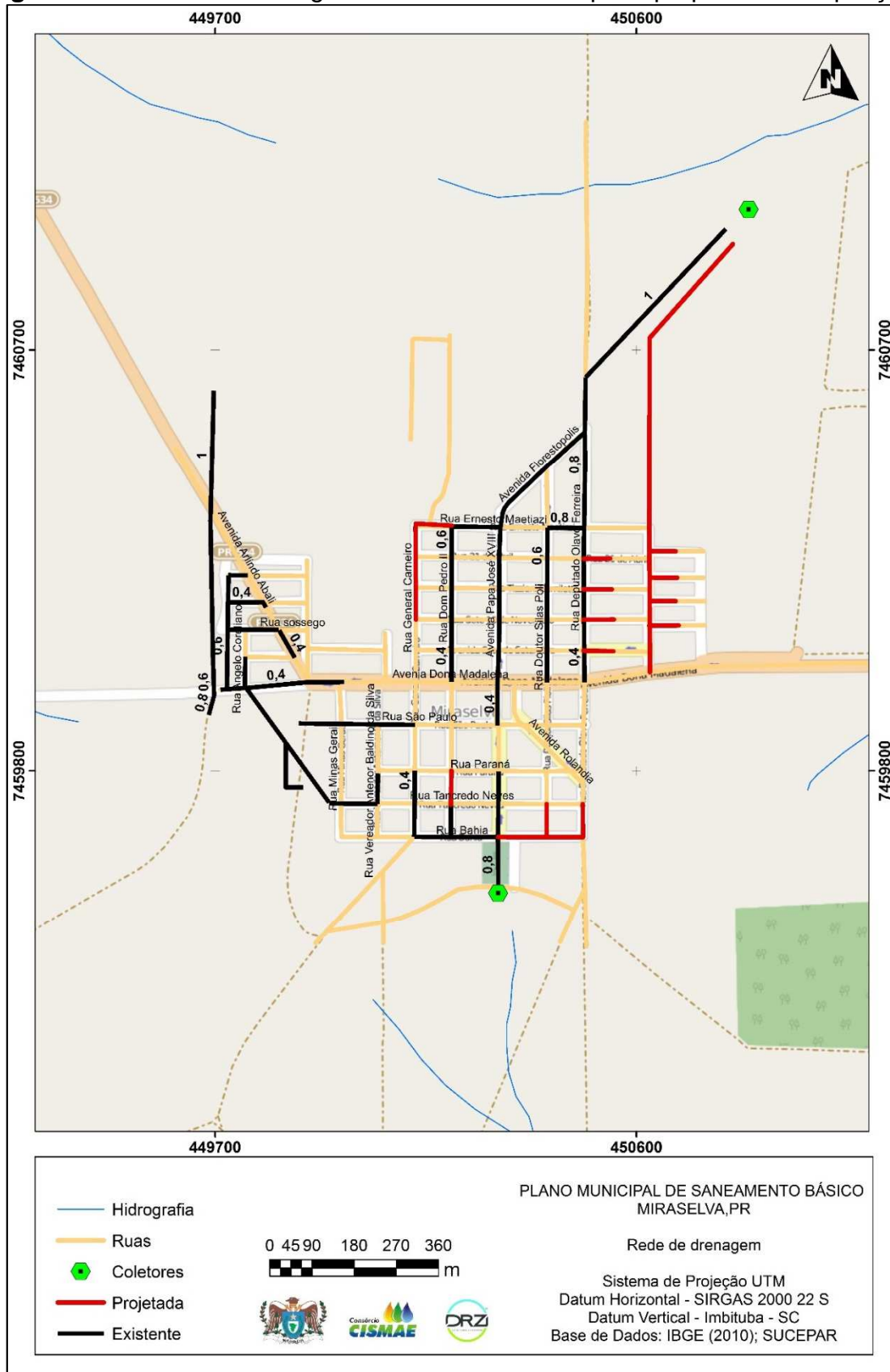
Figura 1.7 – Rede de drenagem existente no município e proposta de ampliação
