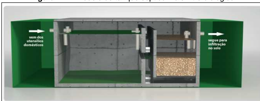
Figura 1.4 – Modelo de tanque séptico mais filtro biológico
