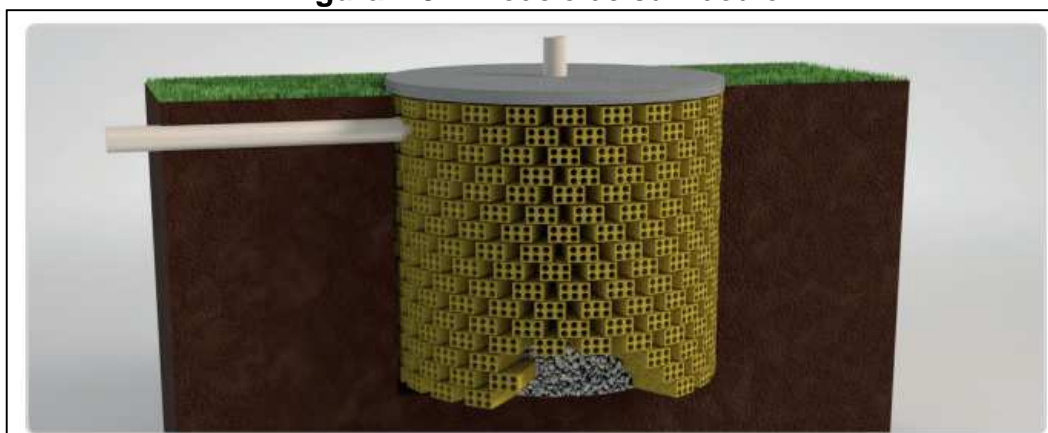
Figura 1.5 – Modelo de sumidouro
