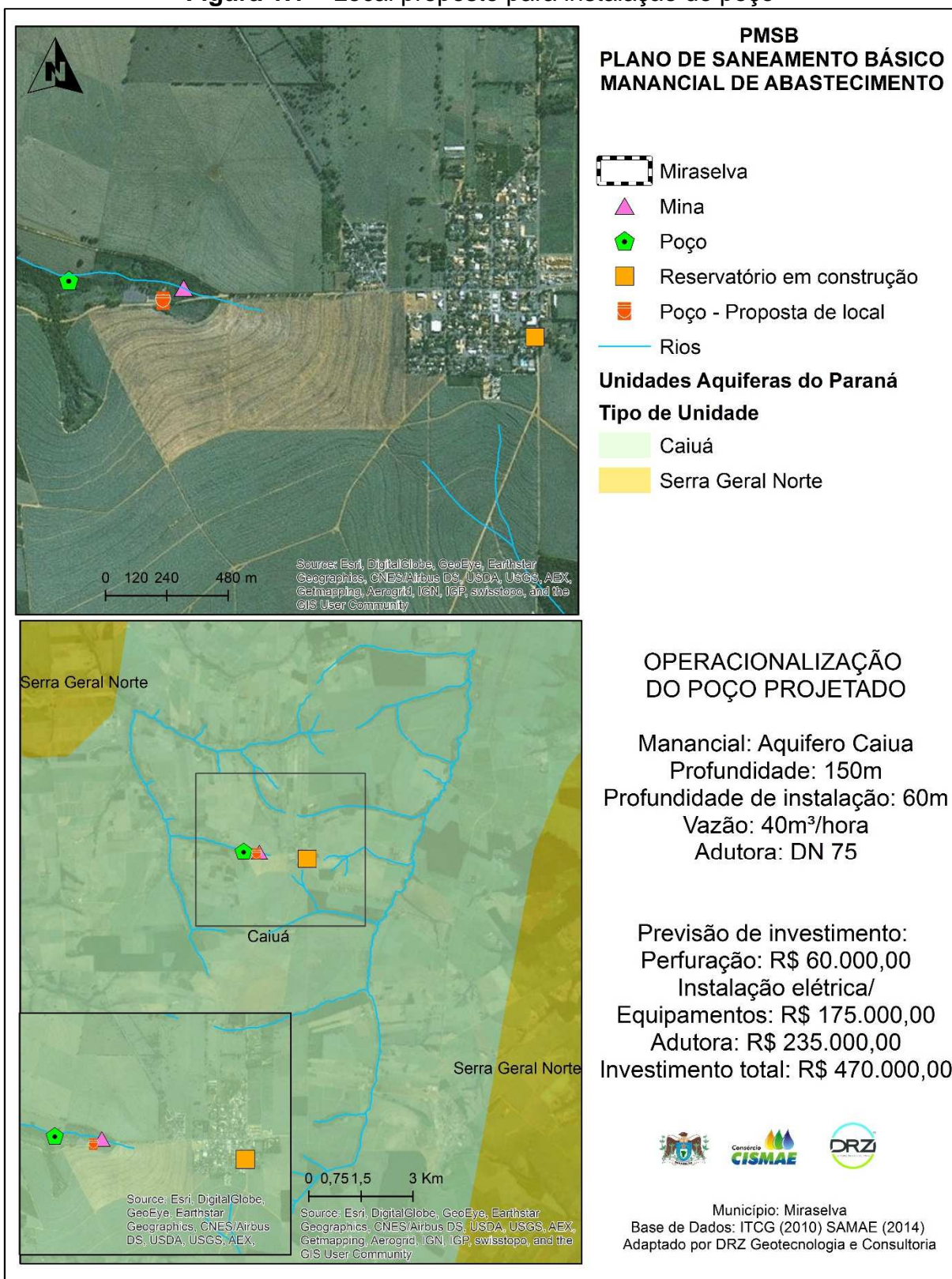
Figura 1.1 – Local proposto para instalação do poço
